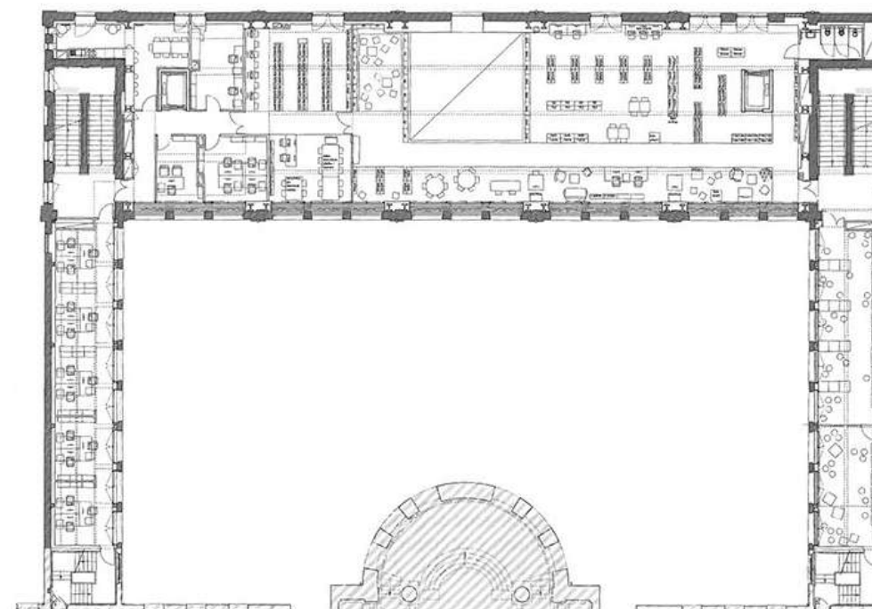
Projet d'aménagement du mobilier au niveau R+1 (© plans Bigoni-Mortemard, architectes).
